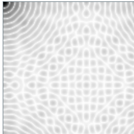
\alpha = 1.4
