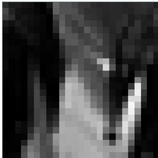
Template
