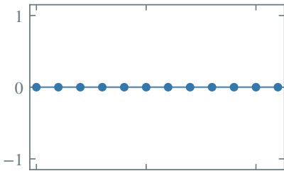
\text{Im } \chi_0
