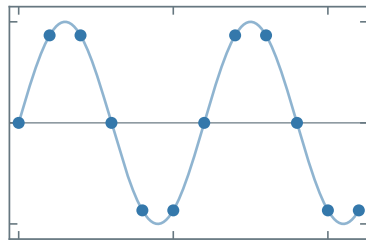
\text{Im } \chi_2
